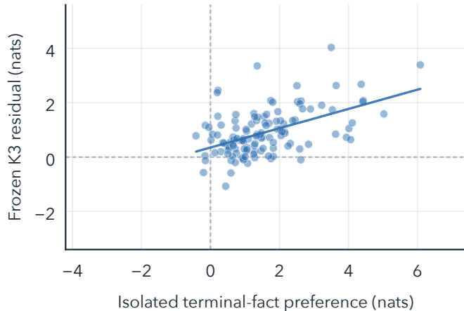
2Wiki
