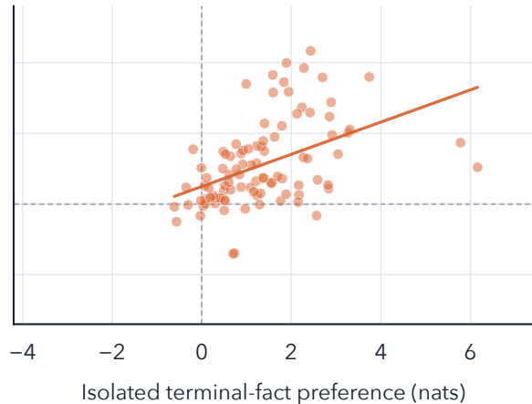
MuSiQue
