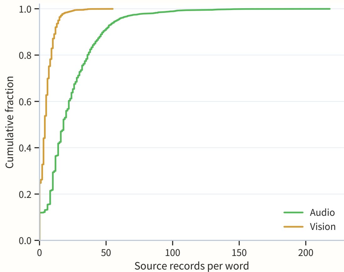
来源密度的累积分布
