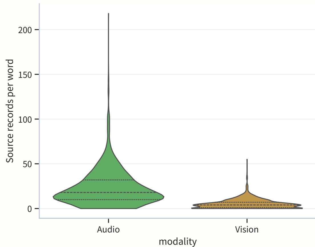
每个词关联的原生来源数
