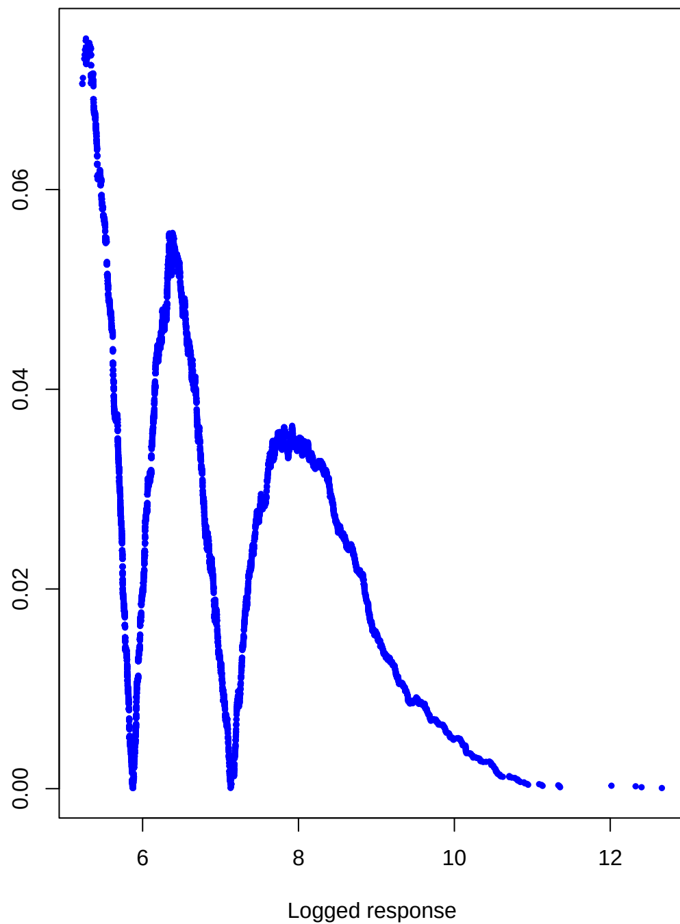
Kolmogorov–Smirnov test
