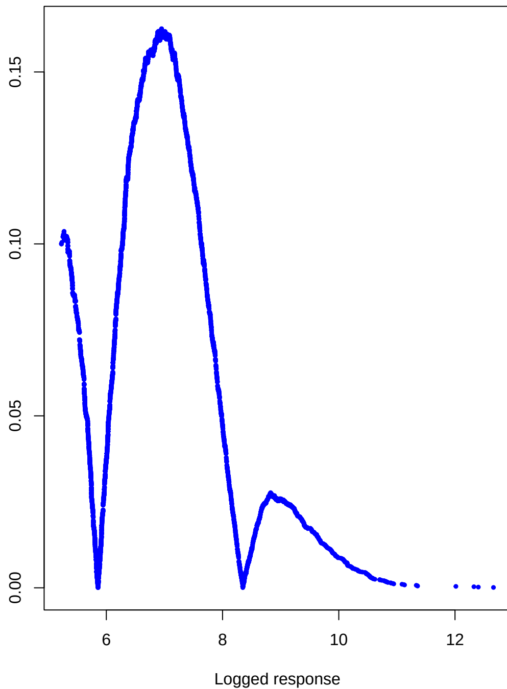
Kolmogorov-Smirnoff test
