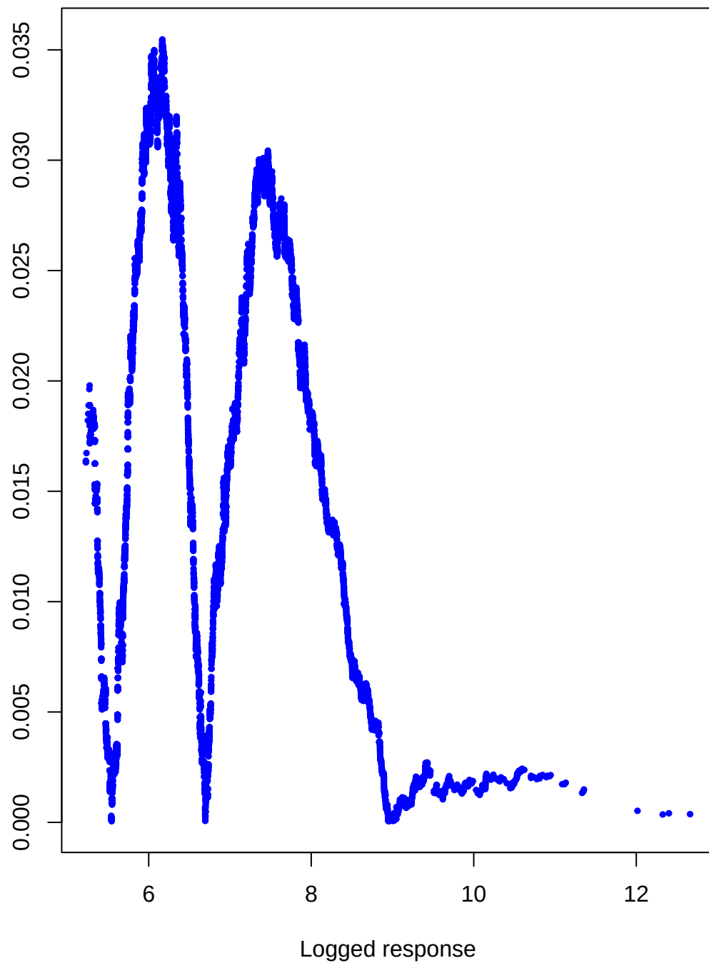
Kolmogorov–Smirnov test
