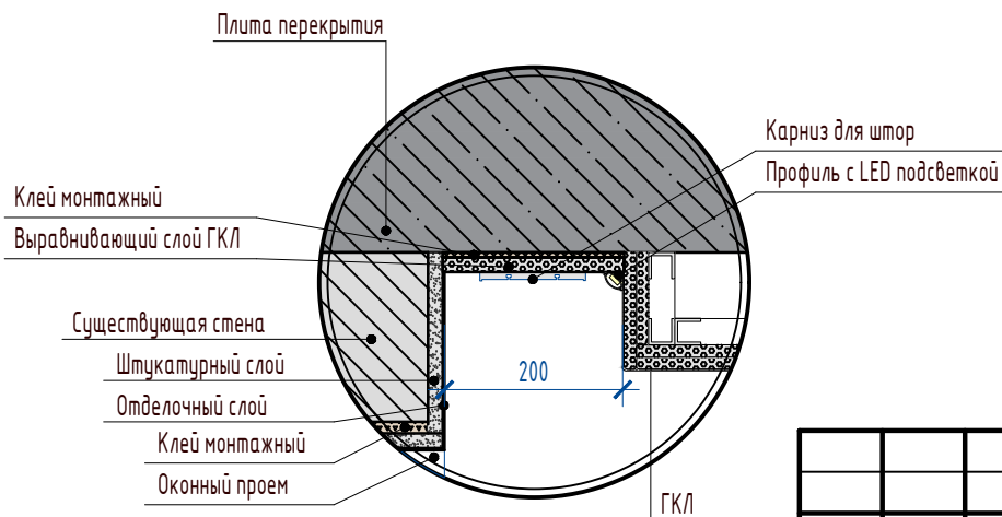
УЗЕЛ Б Формирование ниши для штор с LED подсветкой
