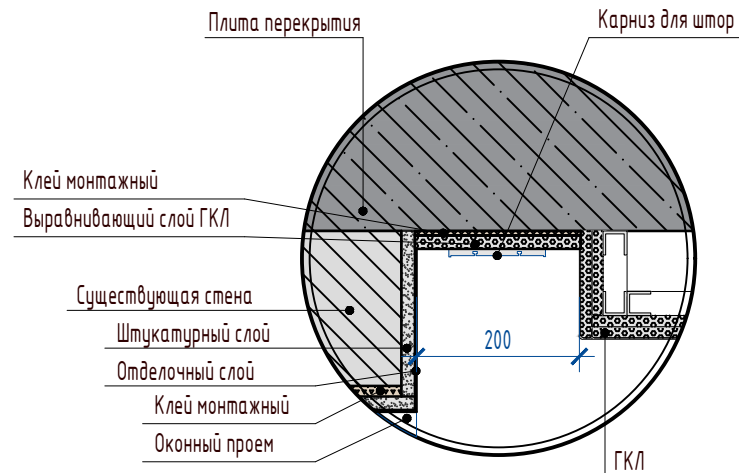
УЗЕЛ А Формирование ниши для штор
