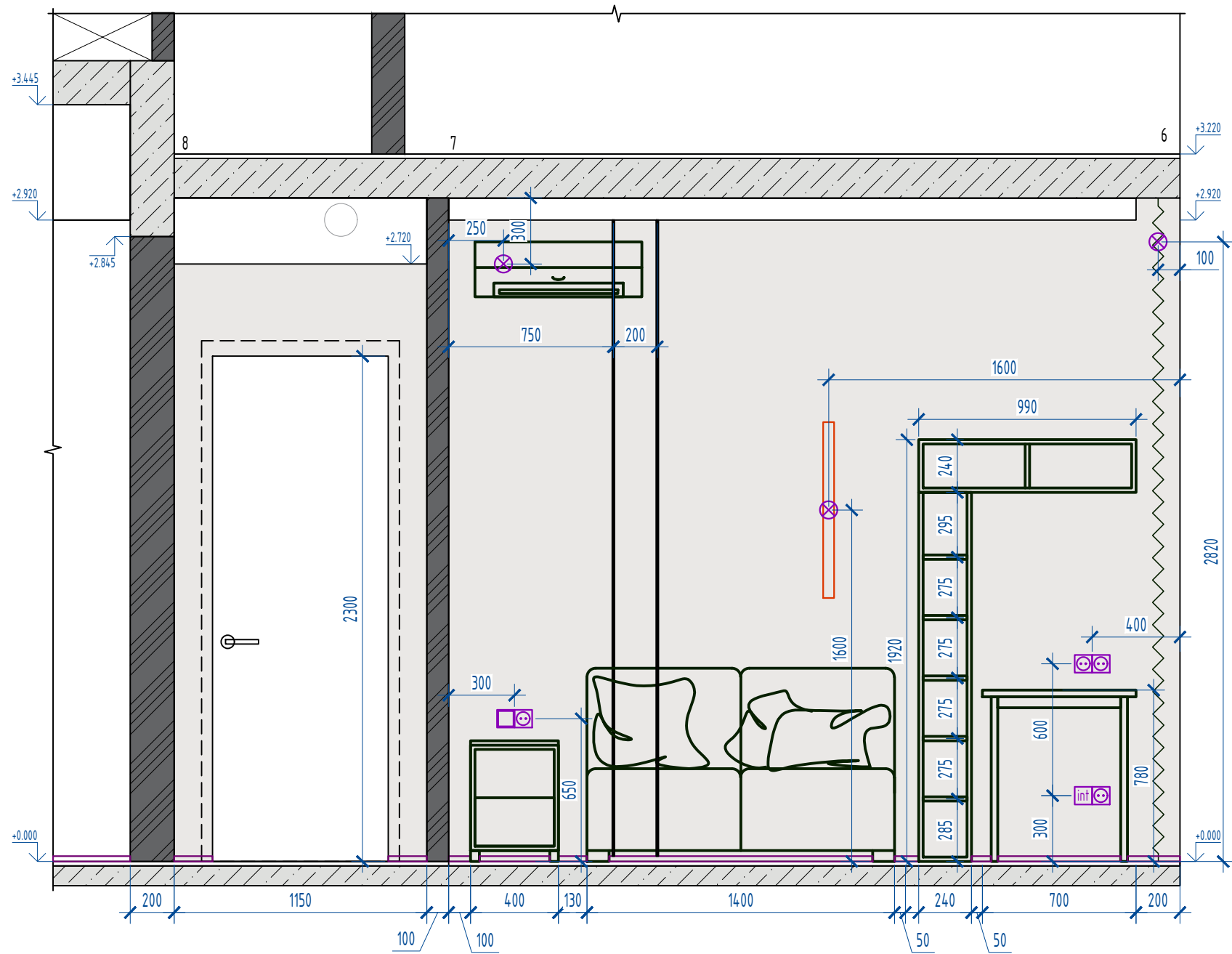
Развертка 8-7-6
