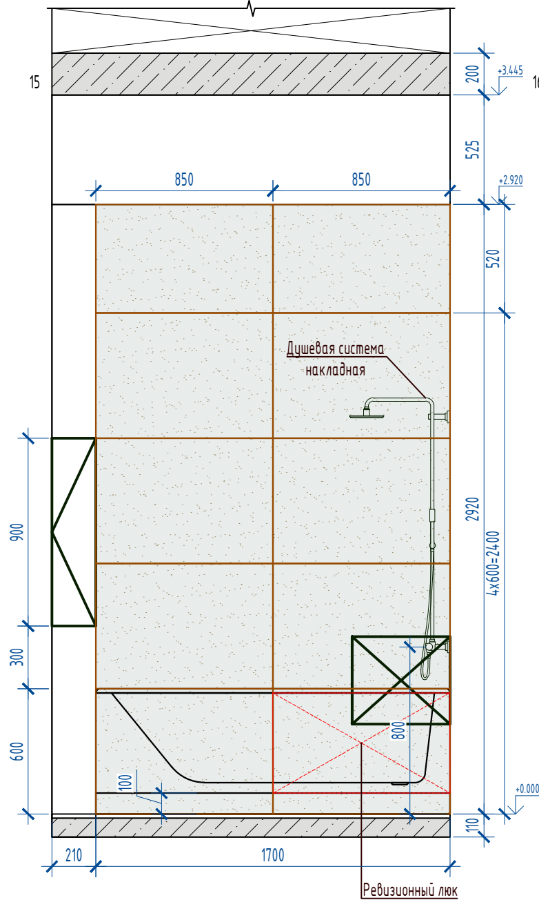
Развертка 15-16
