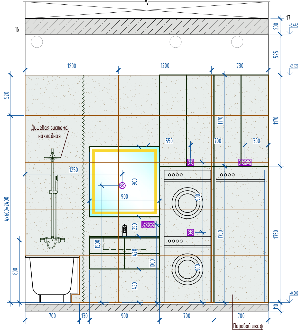
Развертка 16-17
