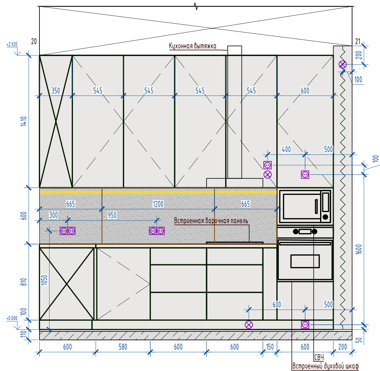
Развертка 20-21
