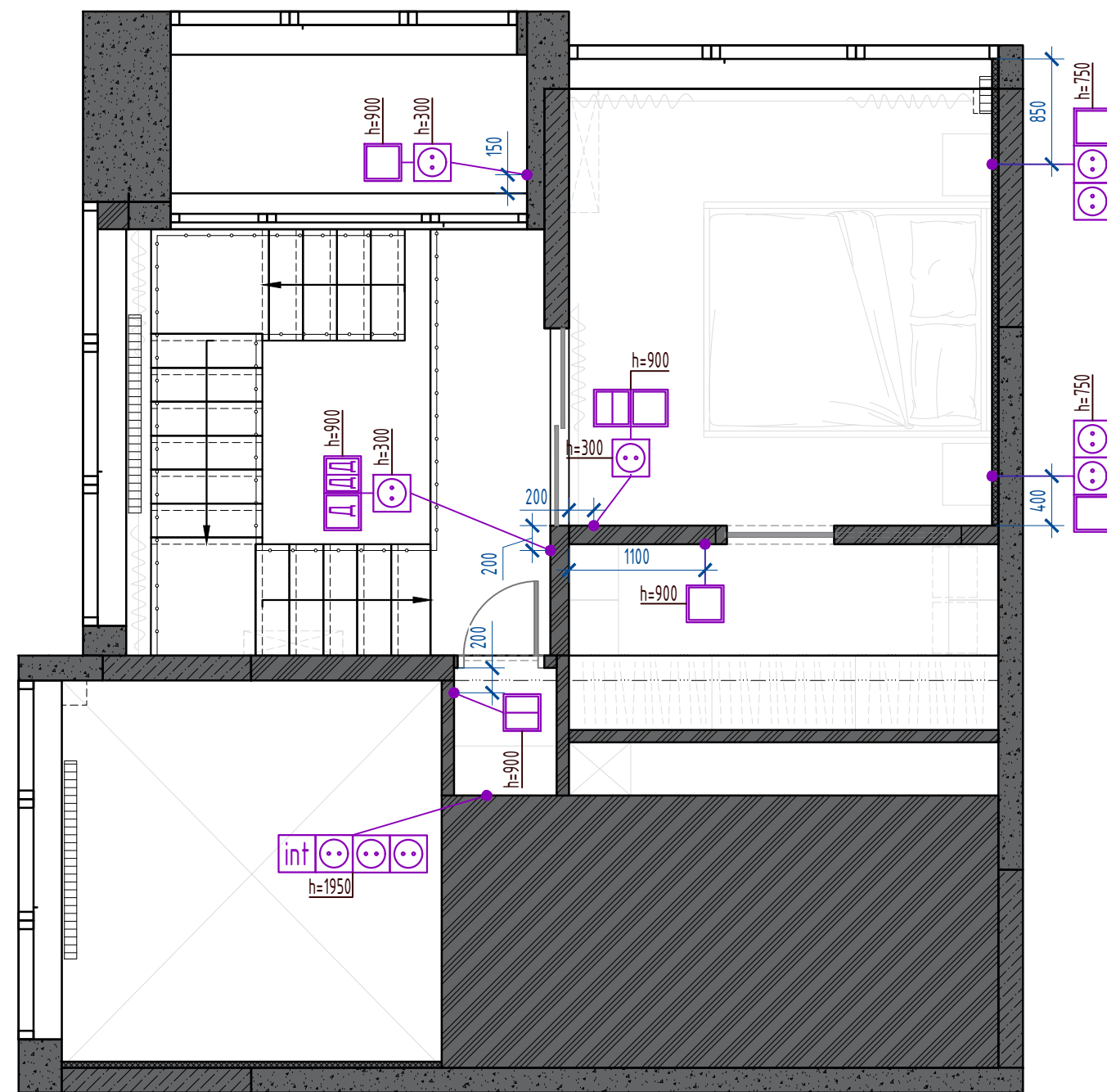
Экспликация электрики
