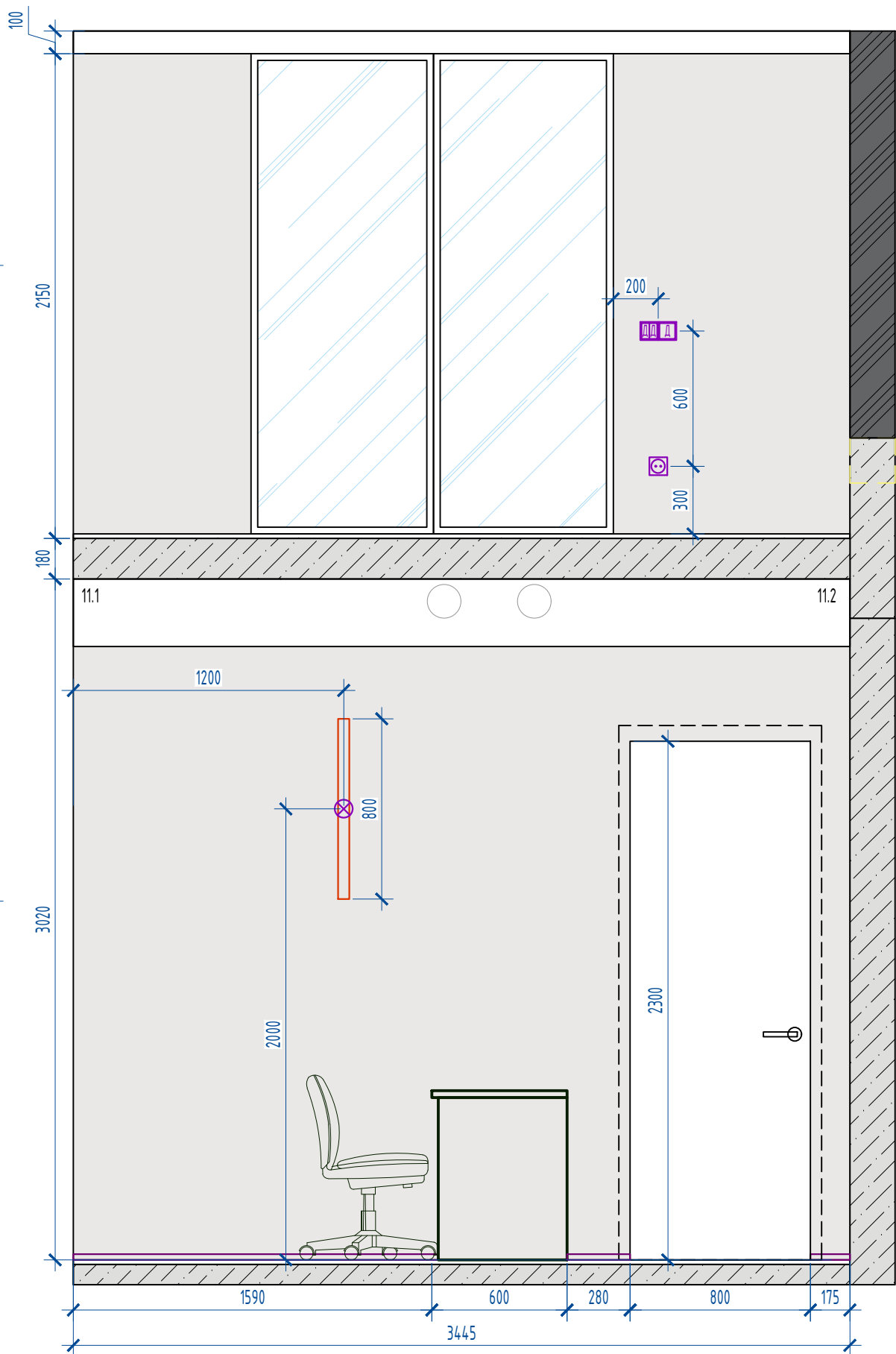
Развертка 11.1-11.2
