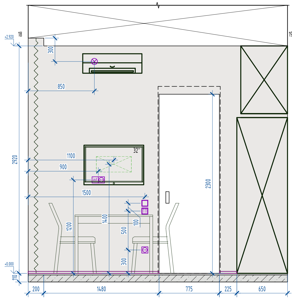
Развертка 18-19
