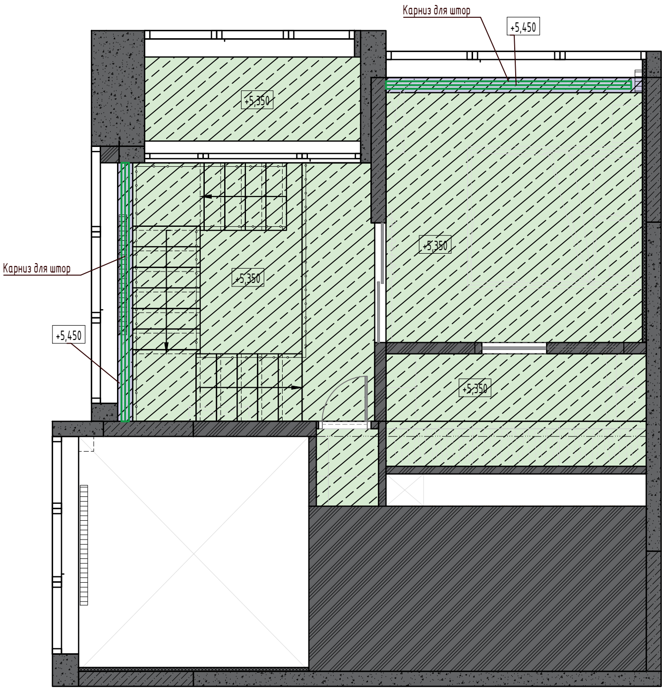
Ведомость отделки потолков
