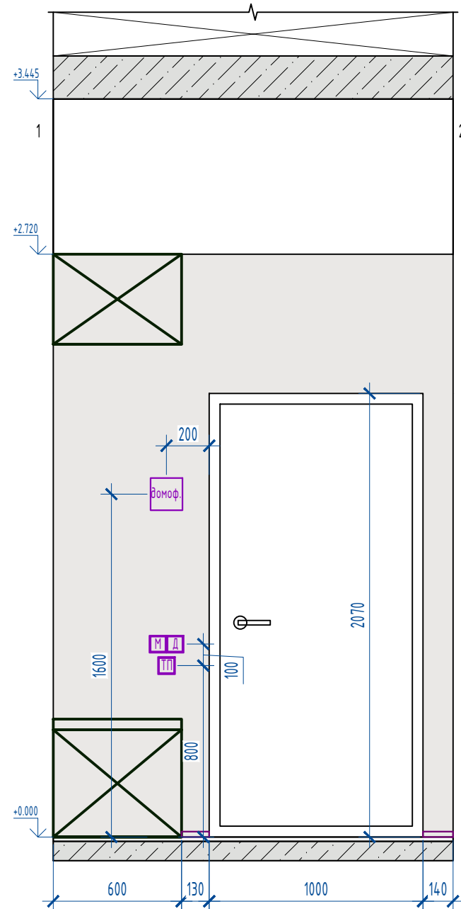
Развертка 1-2
