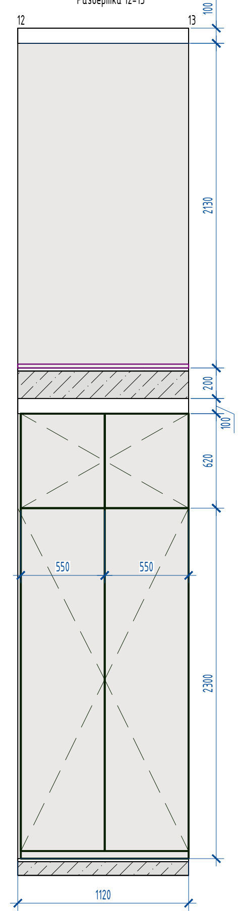
Развертка 12-13
