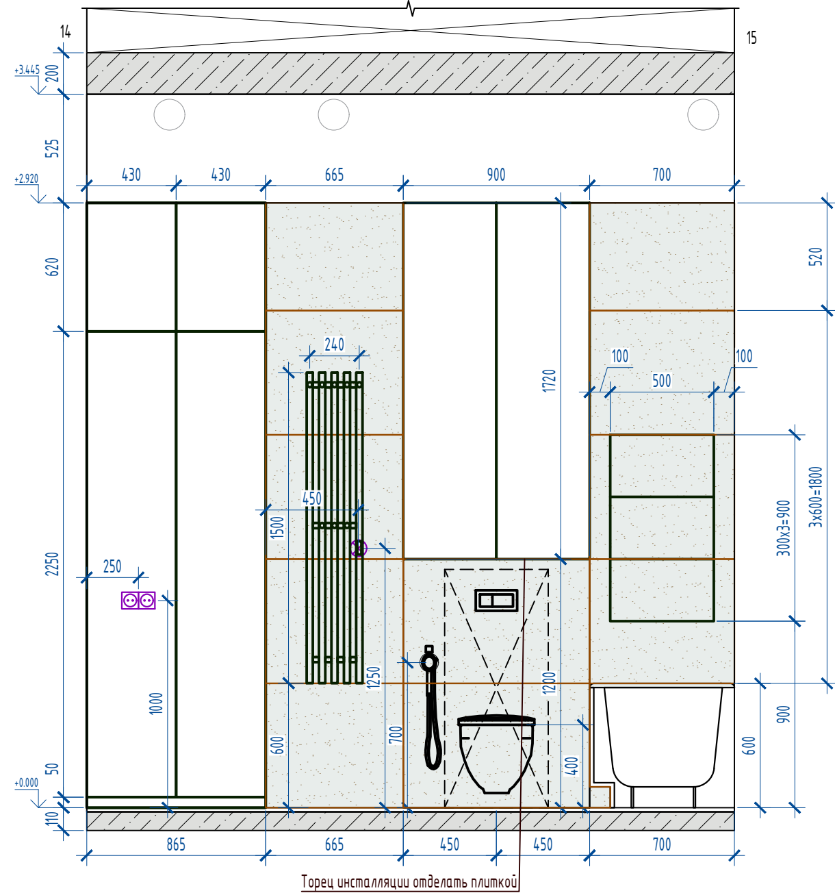
Развертка 14-15
