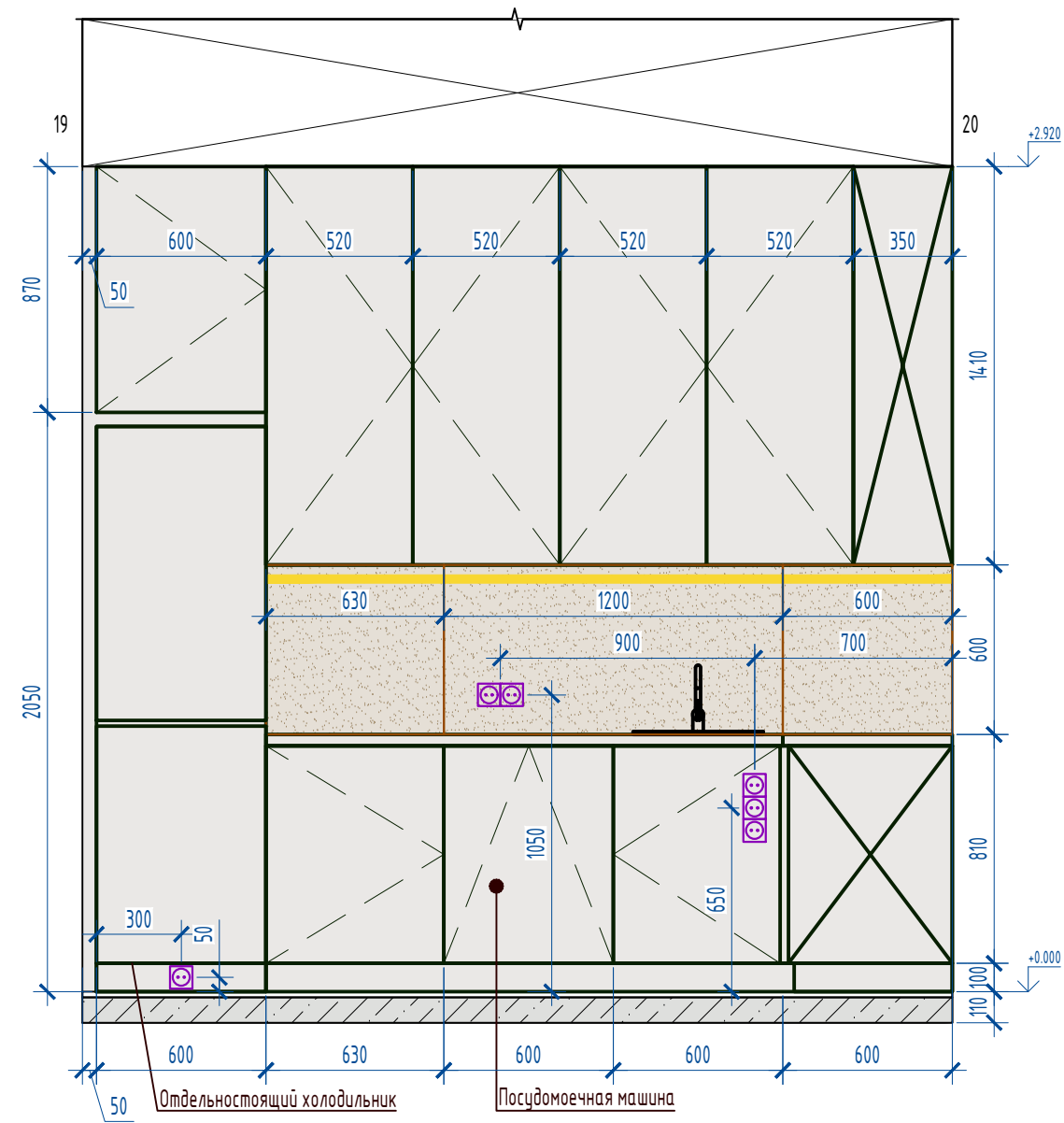
Развертка 19-20
