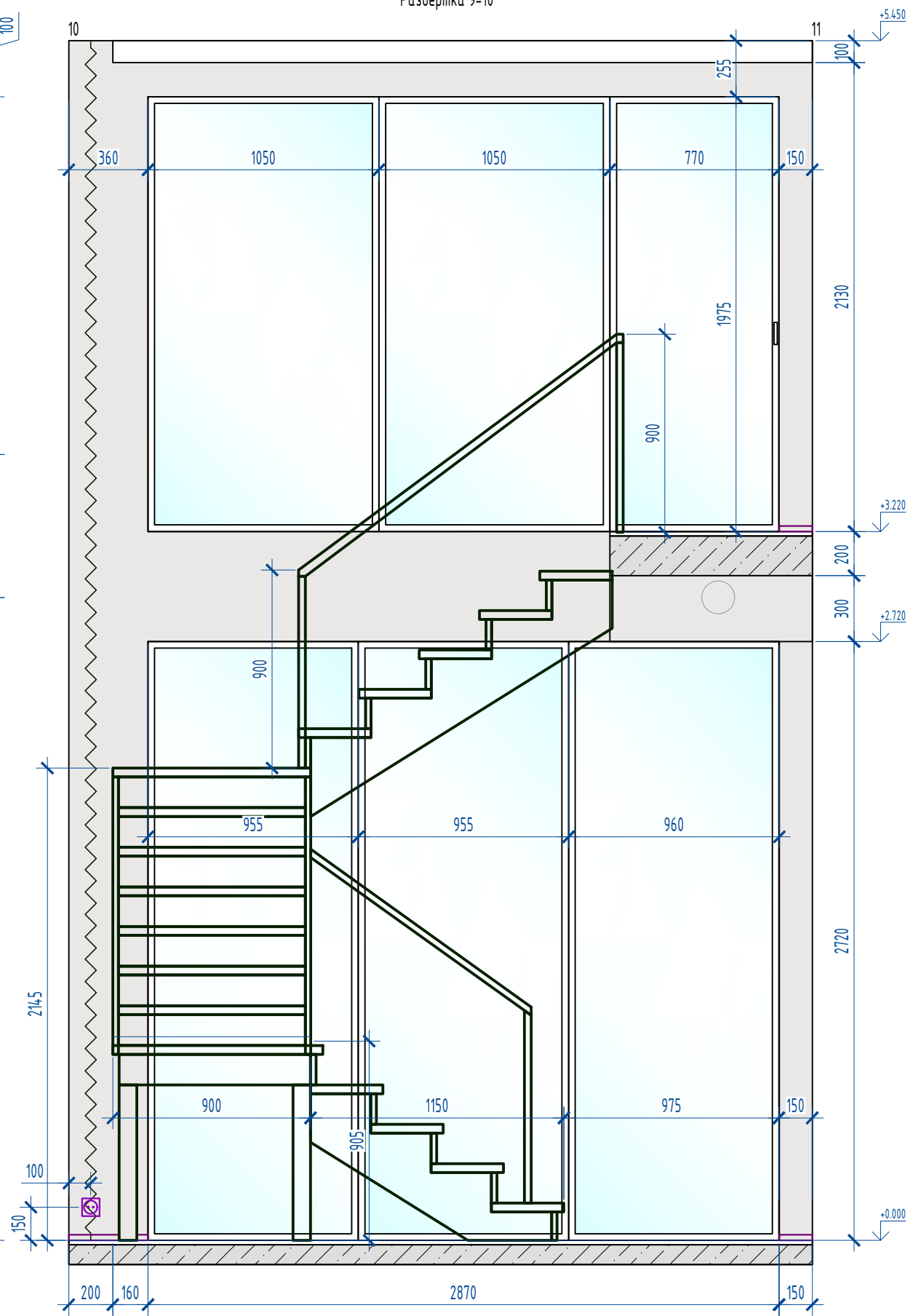
Развертка 9-10
