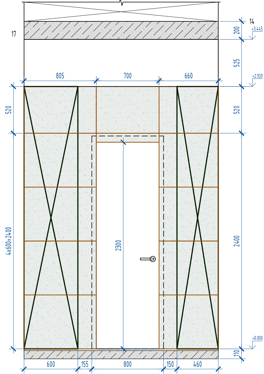
Развертка 17-14
