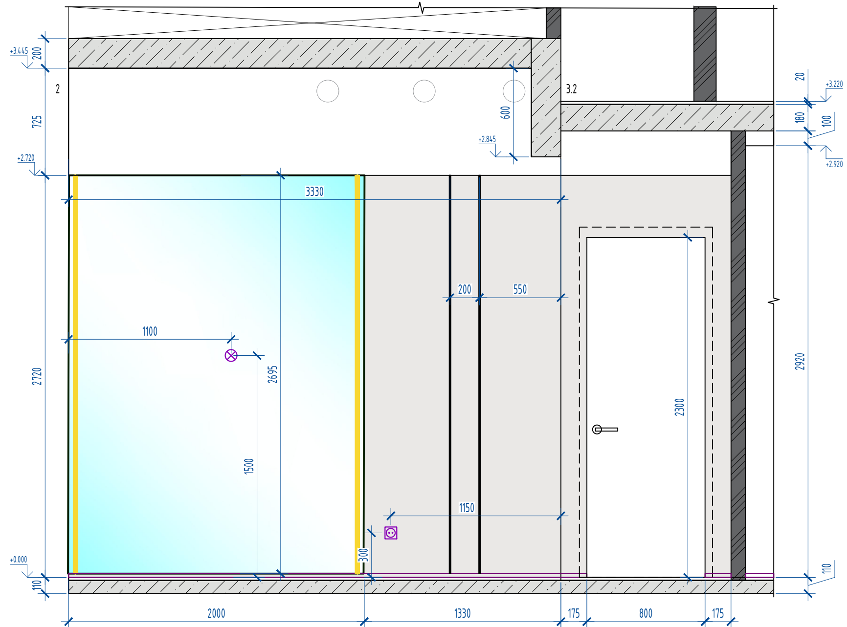
Развертка 2-3.2
