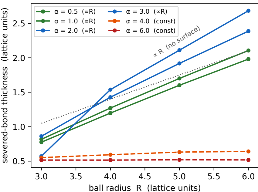
(a) \alpha \leq d : the cut fills the volume; \alpha > d : a membrane
