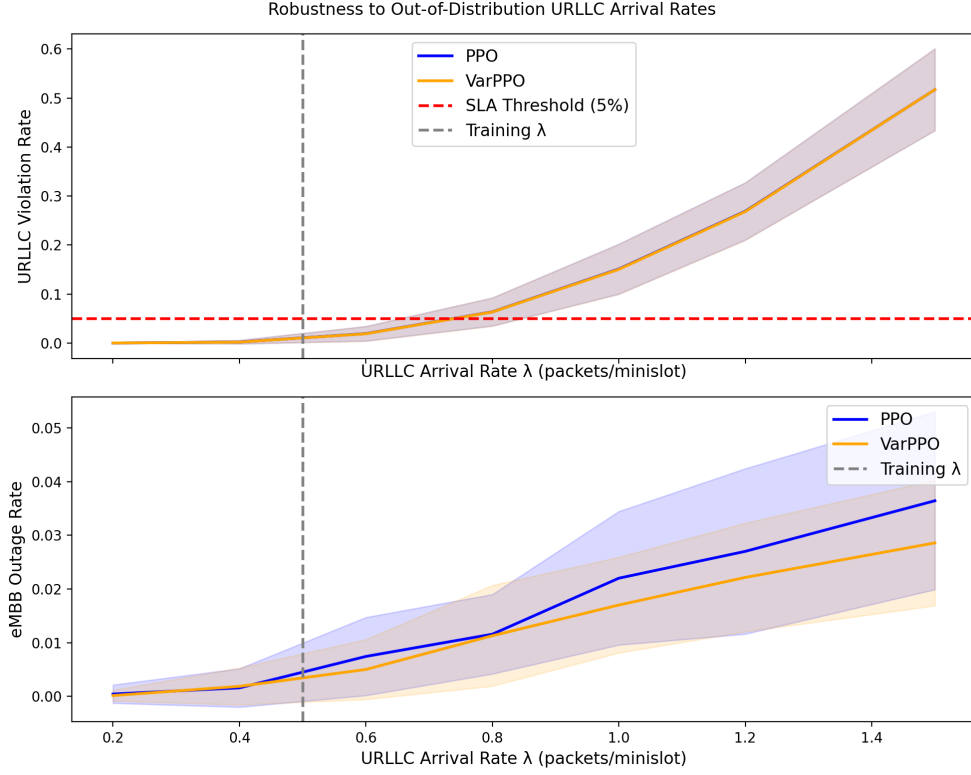
图 4-4 PPO 与 VarPPO 在分布外 URLLC 到达率下的鲁棒性对比
