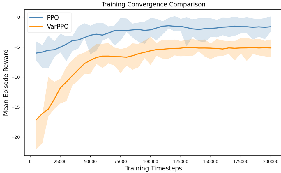
图 4-1 PPO 与方差惩罚 PPO 的训练收敛对比曲线
