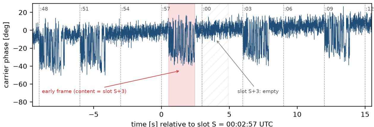
Rys. 1 / Fig. 1. Faza nośnej (IC-705, Wrocław), 27.09.2026 00:02:48–00:03:12 UTC. Zwykłe ramki zaczynają się na granicach slotów (:48, :51, :03, :09). W slotcie :57 przez 0,524 s nie ma modulacji, po czym nadana zostaje ramka z czasem 00:03:00; slot :00 jest pusty. / Carrier phase; regular frames start at slot boundaries, the frame for 00:03:00 starts 0.524 s into slot :57, slot :00 is empty.
