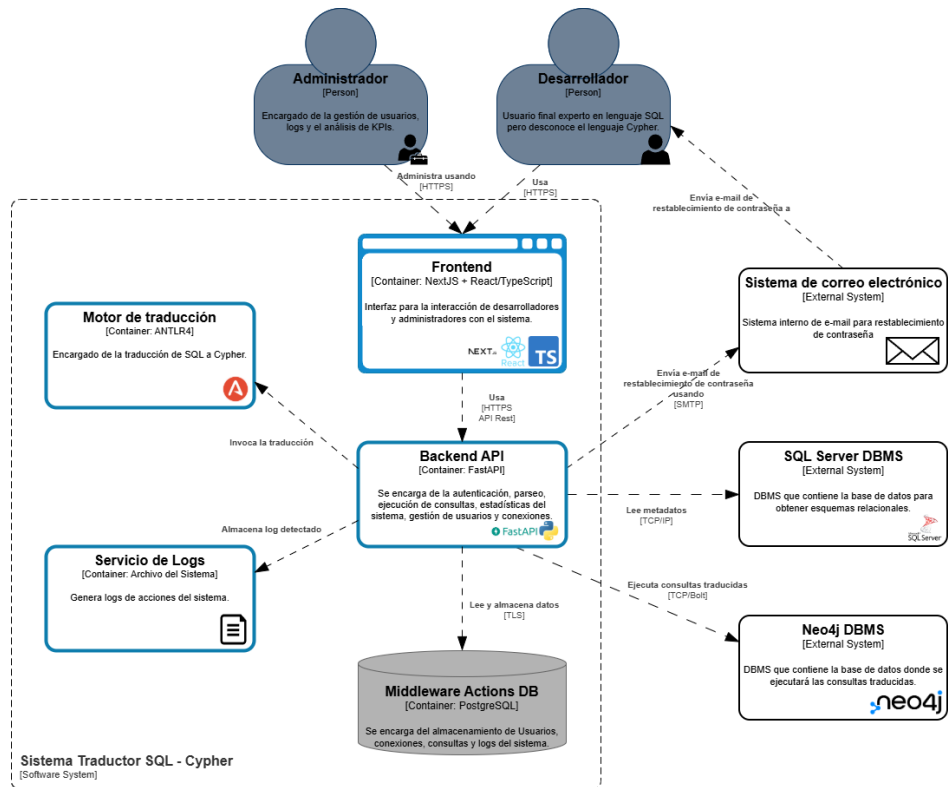
Figura 2.3: Diagrama de contenedores del sistema.
