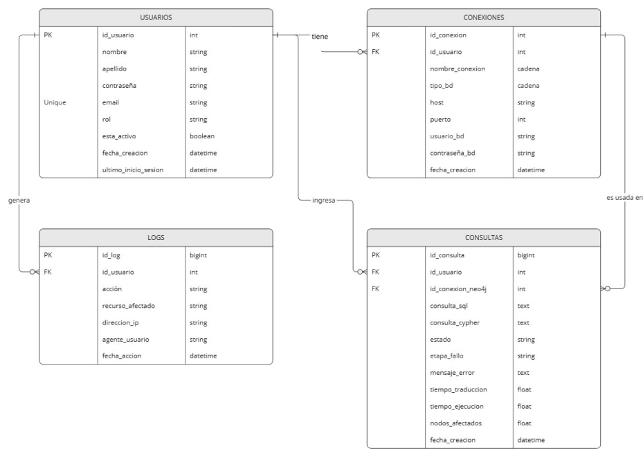
Figura 2.4: Diagrama de base de datos del sistema.
