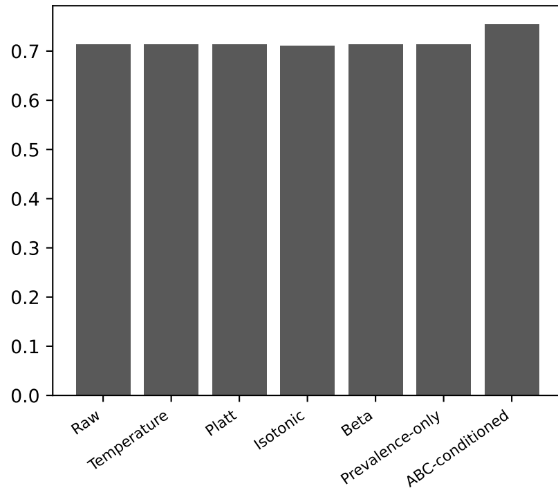
AUC
