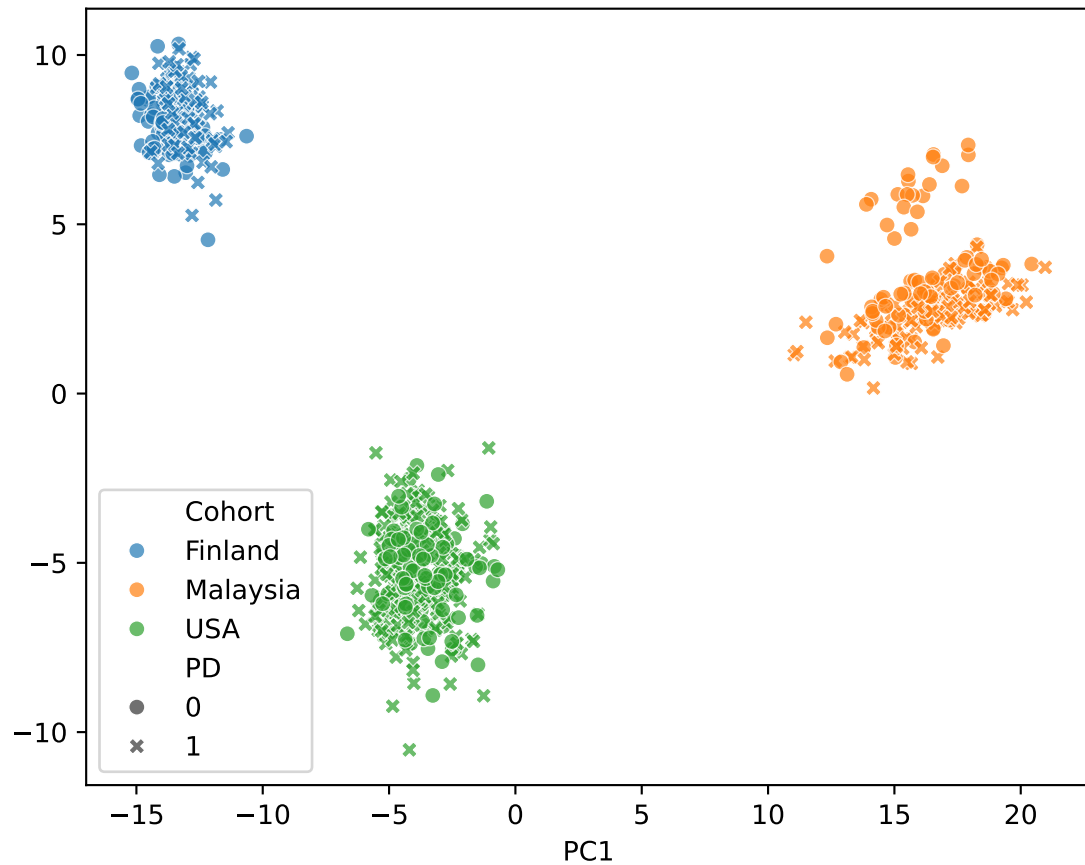
PCA Raw CLR
