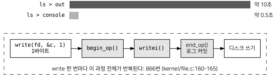
그림 9. 같은 866바이트를 쓰는 데 걸린 시간과 그 이유. ls 는 printf 로 한 글자씩 쓰므로 write 가 866번 불린다. 파일에 쓸 때는 그 때마다 로그 트랜잭션이 열리고 디스크에 커밋된다.
