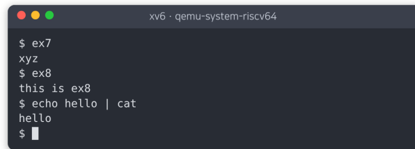
tmux 캡처. ex7 (혼자 쓰고 읽기), ex8 (자식이 쓰고 부모가 읽기), 셸의 파이프.
