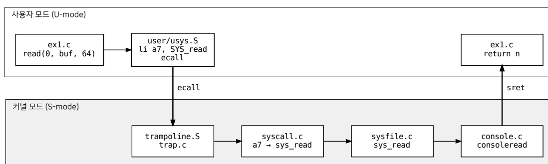
그림 2. read(0, buf, 64) 한 번이 지나가는 길. 사용자 모드에서 ecall 로 들어가 커널을 거쳐 sret 으로 돌아온다. 가운데 단계(트랩펄린, 트랩 처리)는 강의 6에서 다룬다.
