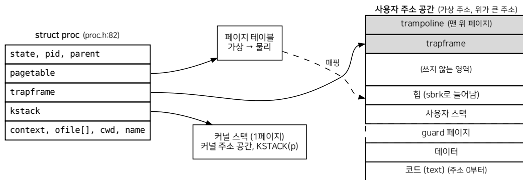
그림 4. struct proc과 주소 공간(교재 그림 2.3). 사용자 주소 공간 맨 위에는 트램펄린과 trapframe 페이지가 있고, 스택 아래에는 접근하면 예외가 나는 guard 페이지가 있다(exec.c:87--95).
