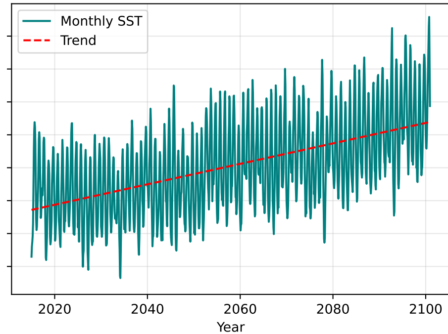
SSP3-7.0
