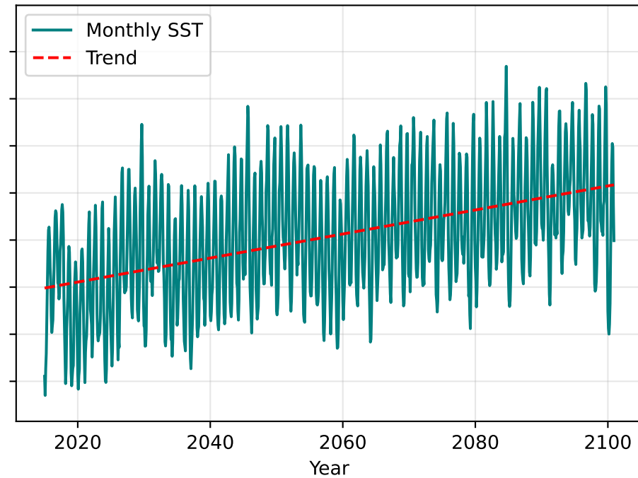
SSP2-4.5
