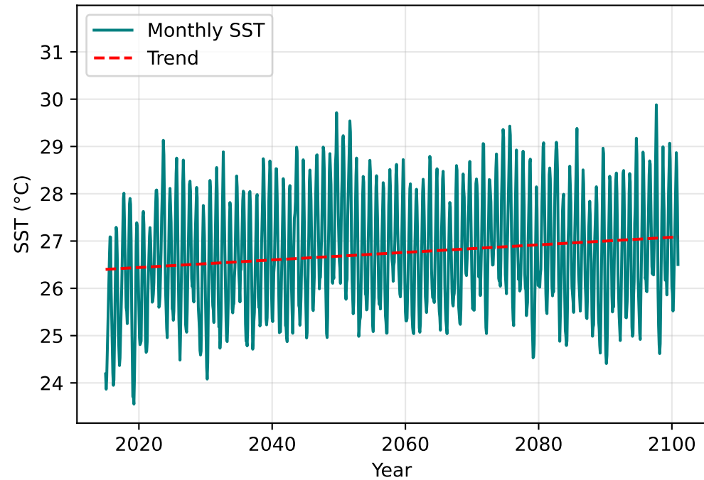
SSP1-2.6
