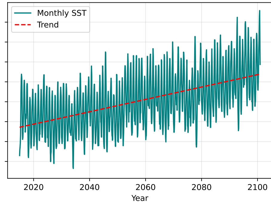
SSP3-7.5
