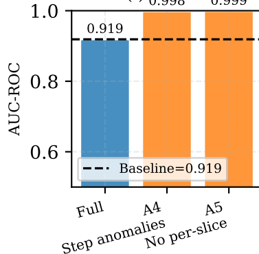
(f) IF AUC
