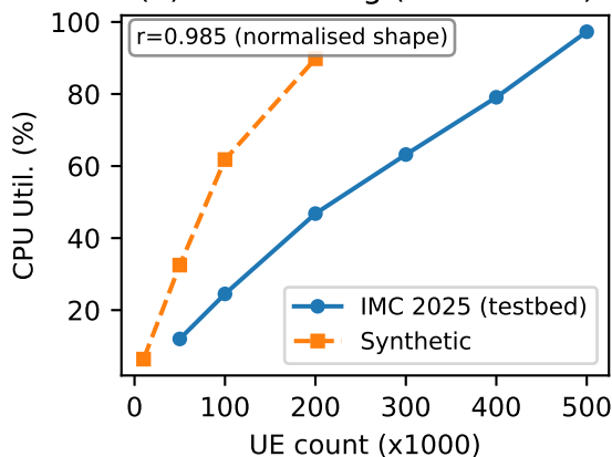
(a) CPU Scaling (absolute %)
