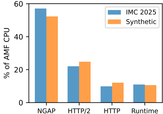
(d) AMF CPU Module Breakdown
