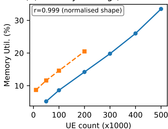
(b) Memory Scaling (absolute %)
