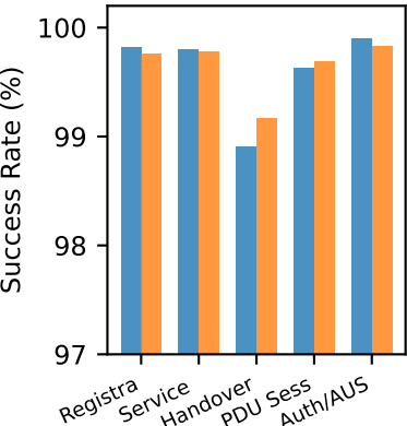
(d) Procedure Success Rate (absolute — 3GPP structural)
