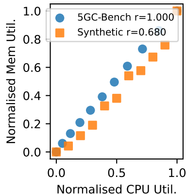
(d) CPU vs. Memory Correlation
