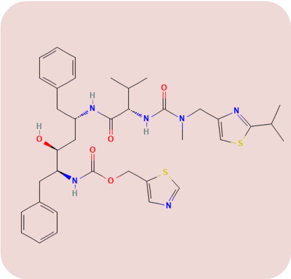
Ritonavir
