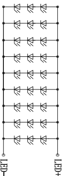
LED电路图:
