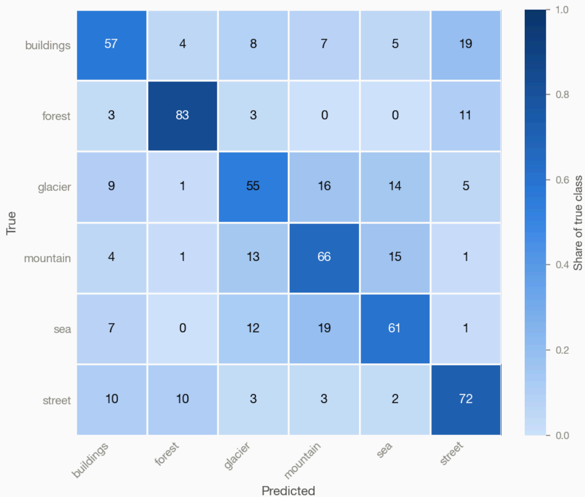
Simple CNN
