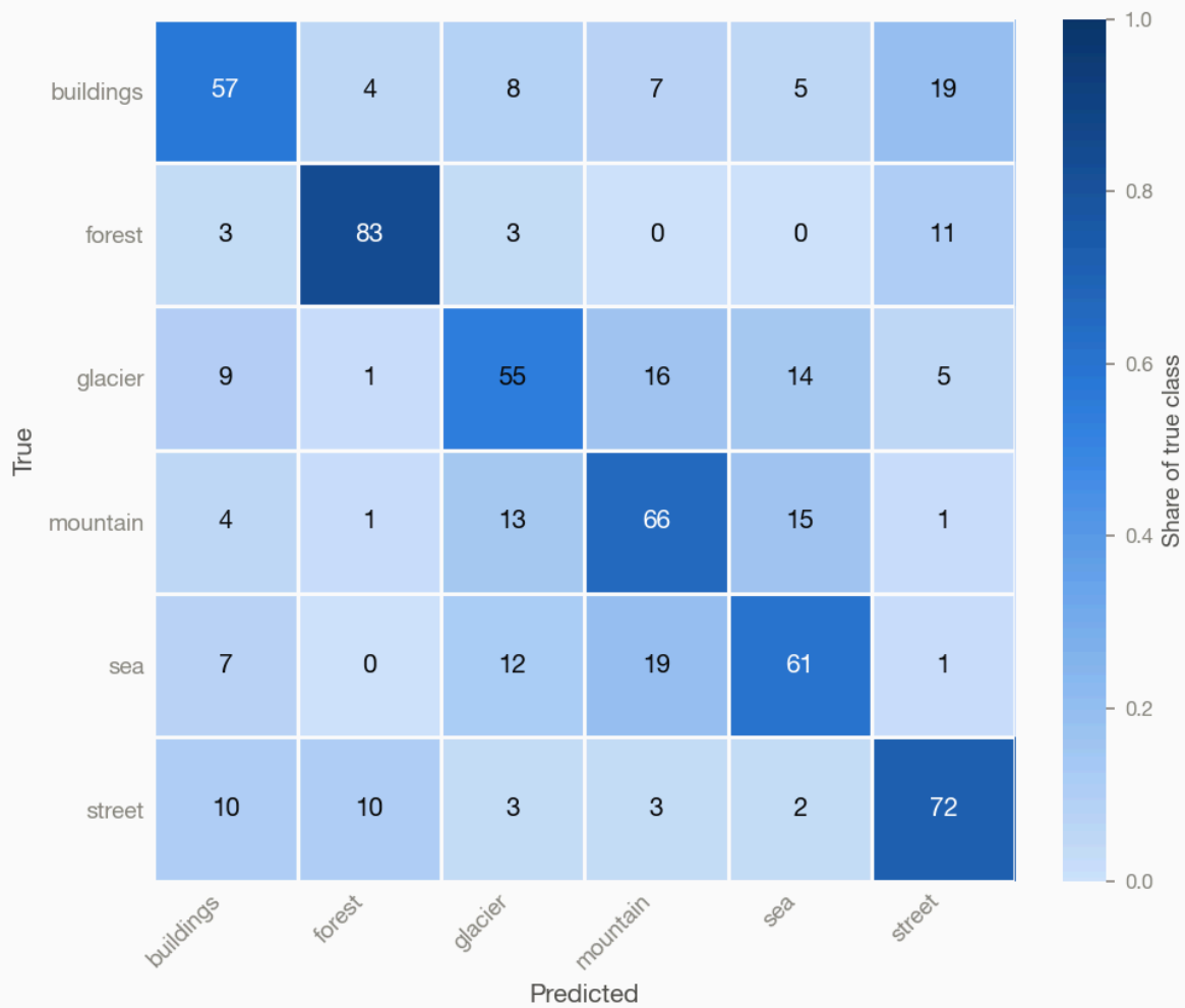
Simple CNN
