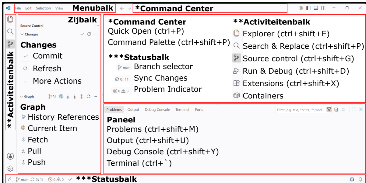
Figuur 1: Benaming van de belangrijkste schermonderdelen in VS Code met betrekking tot Git
