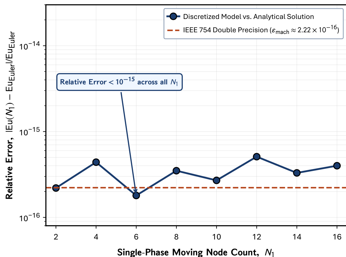
(d) Mesh Independence &amp; Machine Precision
