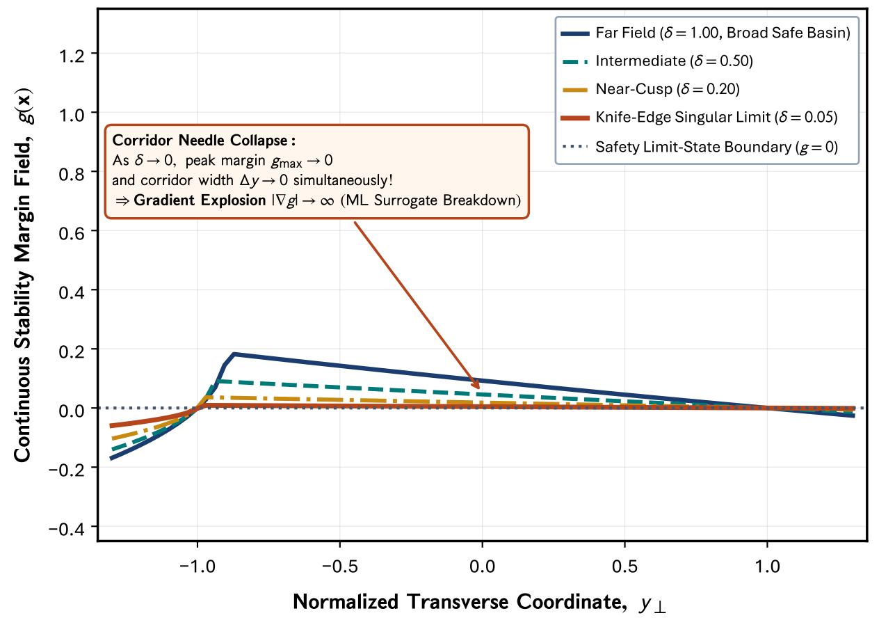
(d) Transverse Stability Margin Field Compression
