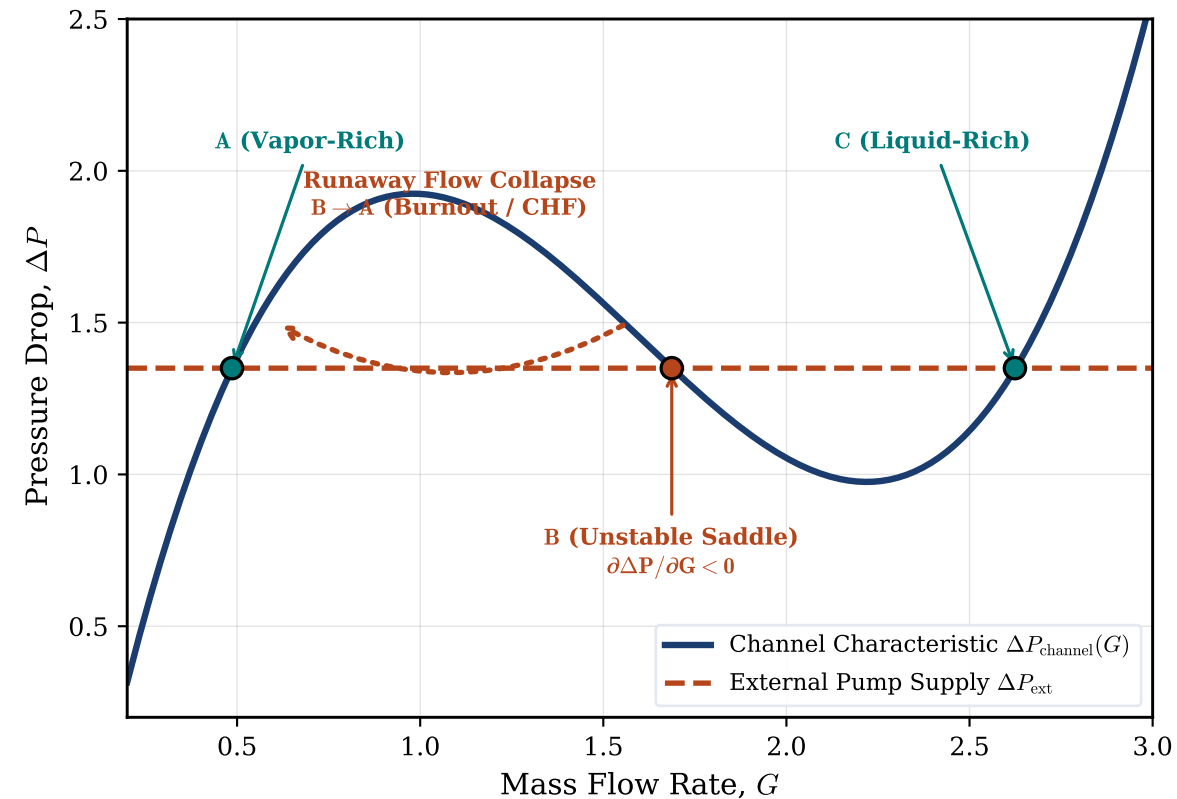
(d) Static Ledinegg Instability &amp; Flow Excursion
