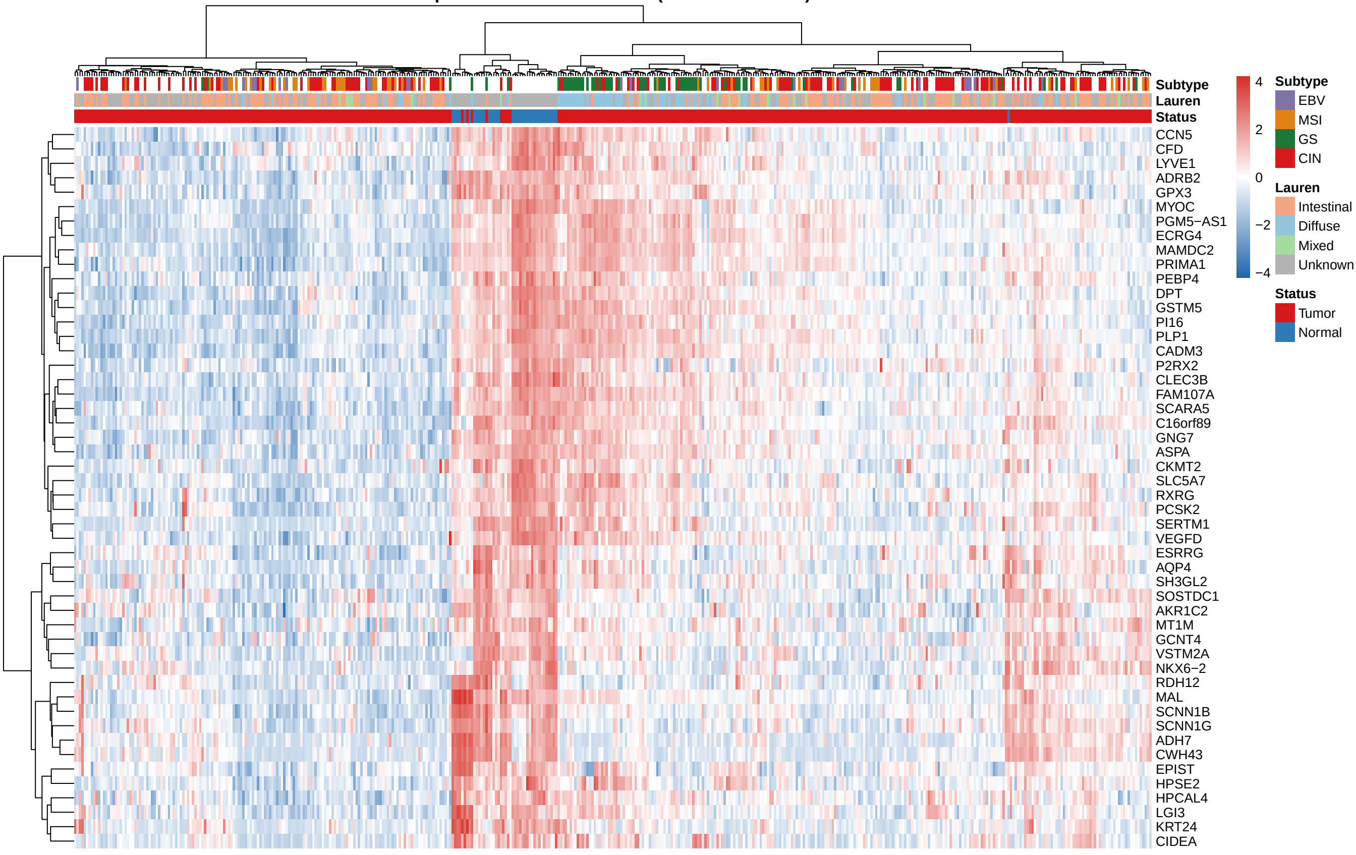
Top 50 DEGs ... TCGA-STAD (Tumor vs Normal)
