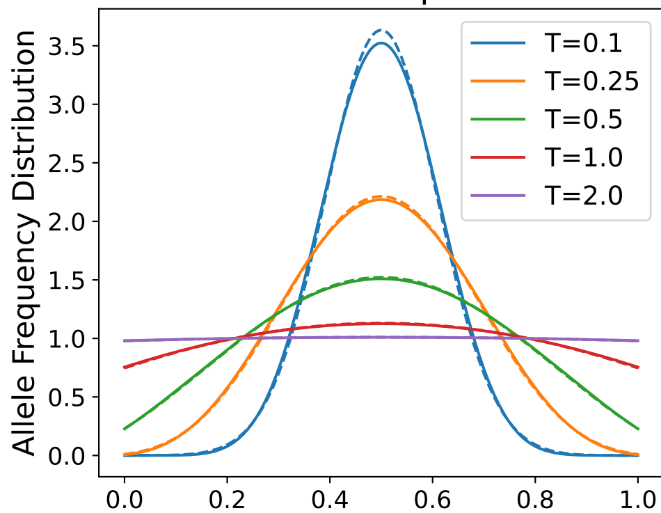
Autotetraploid
