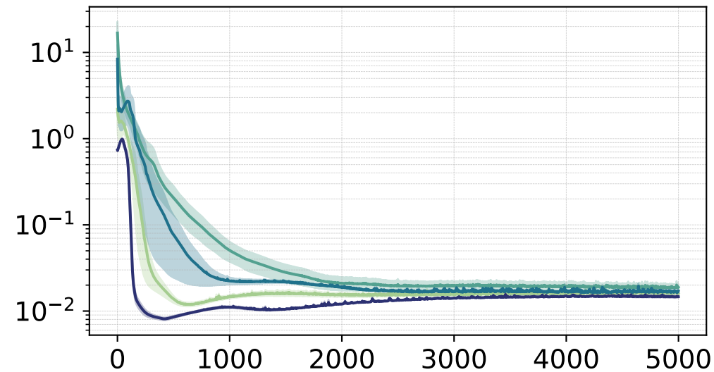
Allen-Cahn
