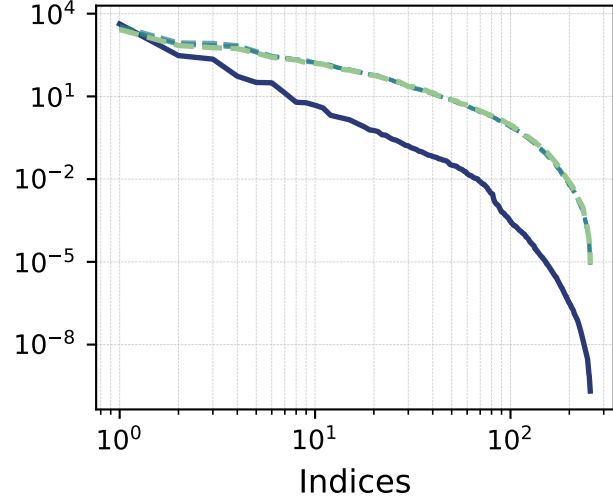
Power-Law
