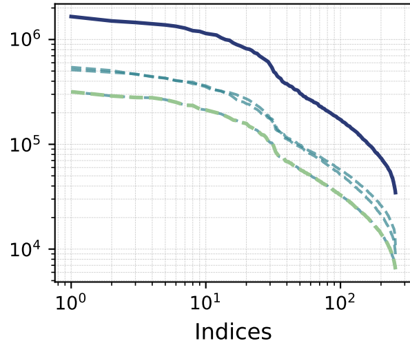
LeCun
