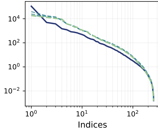
Glorot
