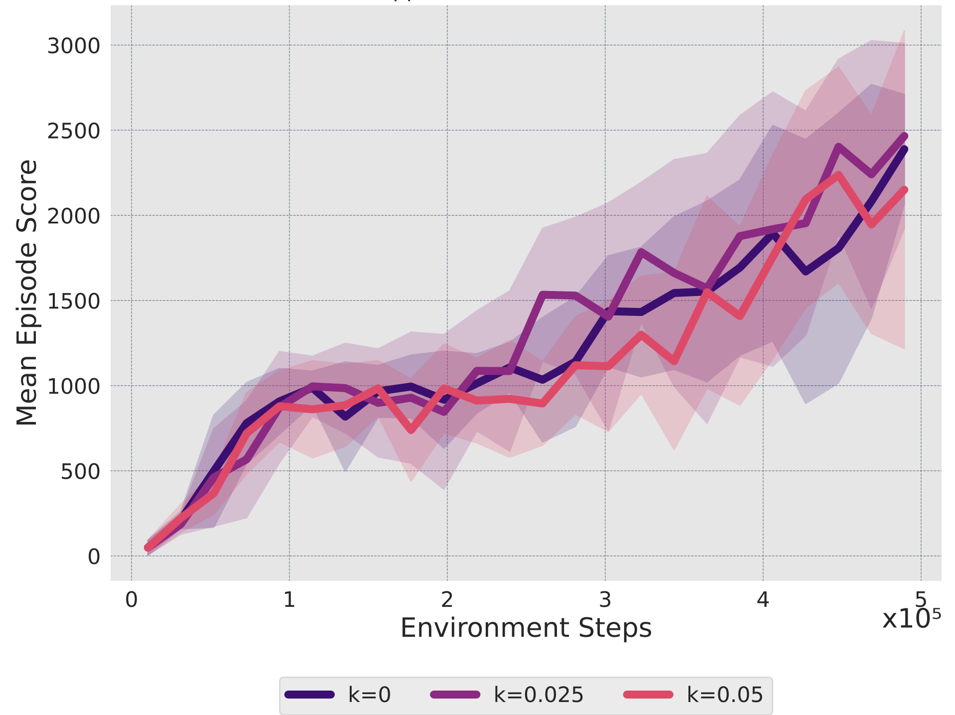
Hopper-v5 (Control Cost - 10x)
