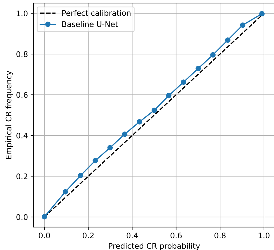
F814W - Globular Clusters ECE=0.0010
