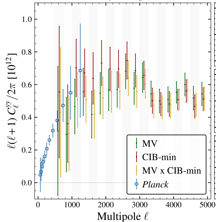
tSZ-only bandpowers
