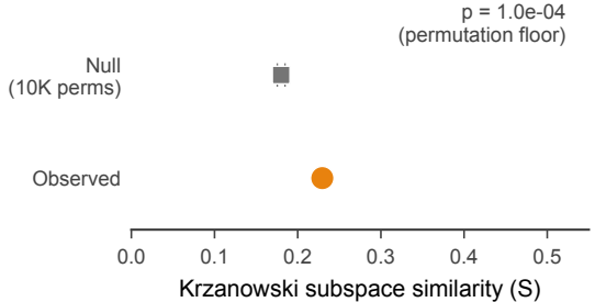
Layer 2: Post-rotation (k=5)
