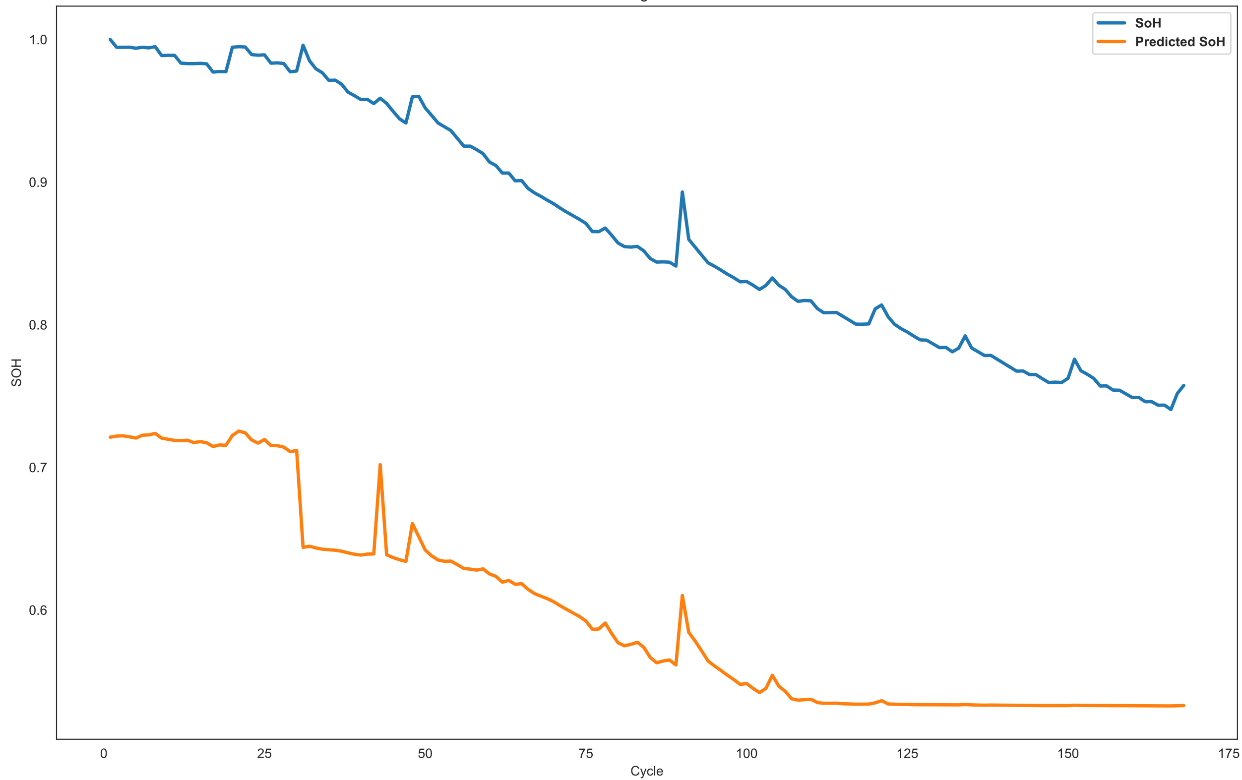
Discharge B0007
