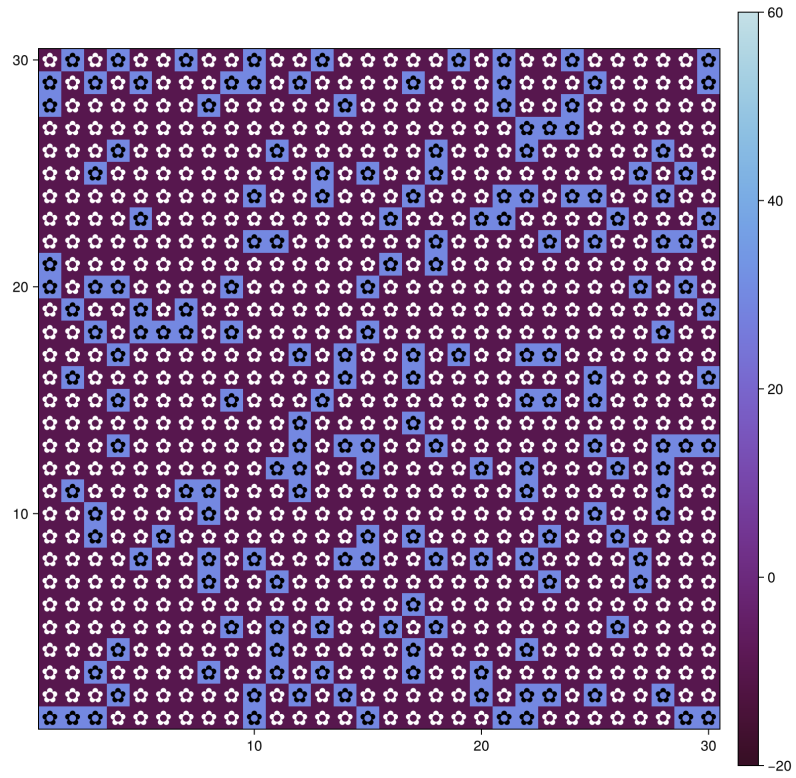
Рисунок 4.32: daisyworld__param.jl
