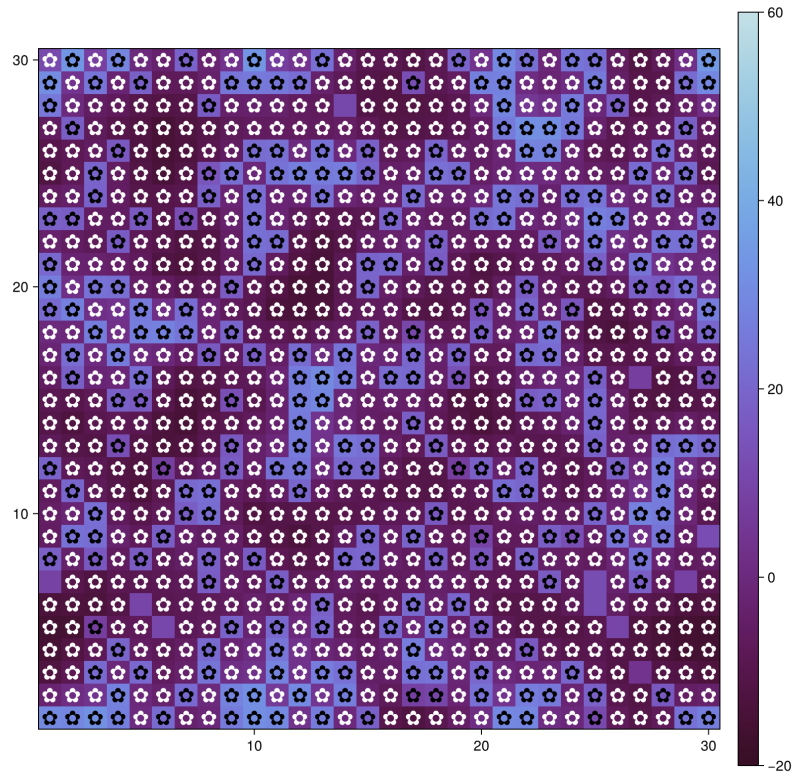
Рисунок 4.33: daisyworld__param.jl
