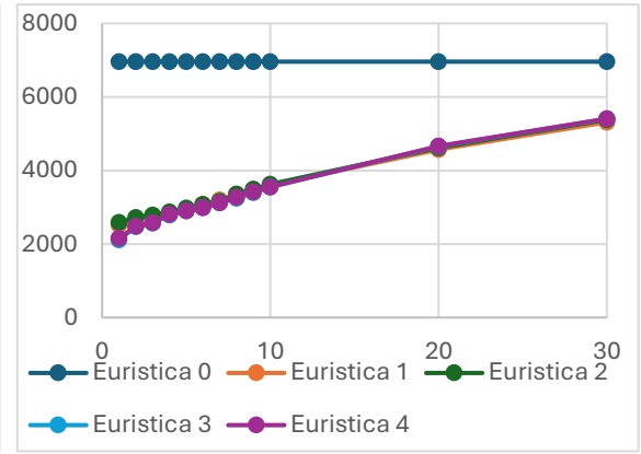
Figura 5.4: n. chiamate ricorsive Petster Hamster network
