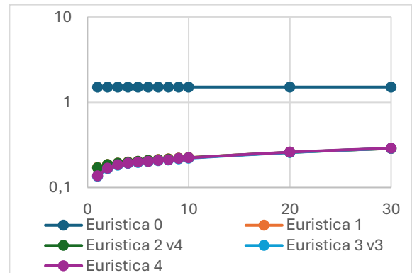
Figura 5.6: n. chiamate ricorsive (milioni) Brightkite
