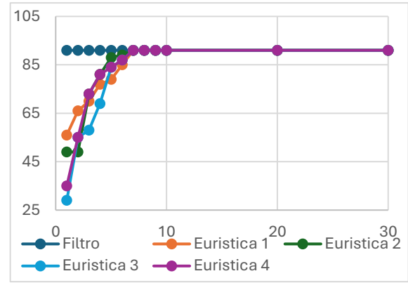
Figura 5.2: n. chiamate ricorsive Zachary Karate Club
