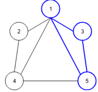
Figura 1.12: clique 1-isolata
