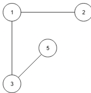
Figura 1.5: sottografo di G_1
