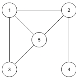
Figura 1.4: grafo G_1
