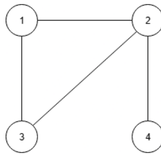
Figura 1.2: grafo non orientato
