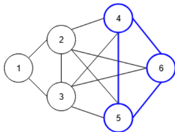
Figura 1.7: clique non massimale
