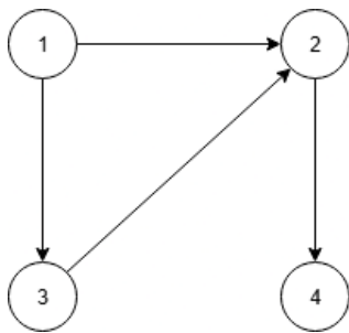
Figura 1.1: grafo orientato
