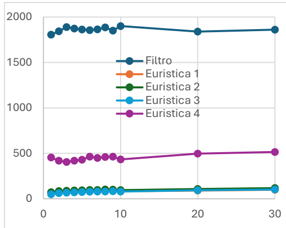
Figura 5.7: tempi di esecuzione (s) AS-Skitter
