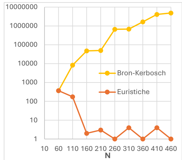
Figura 5.16: n. clique massimali e L -isolate al variare di N , con F , P e L fissi
