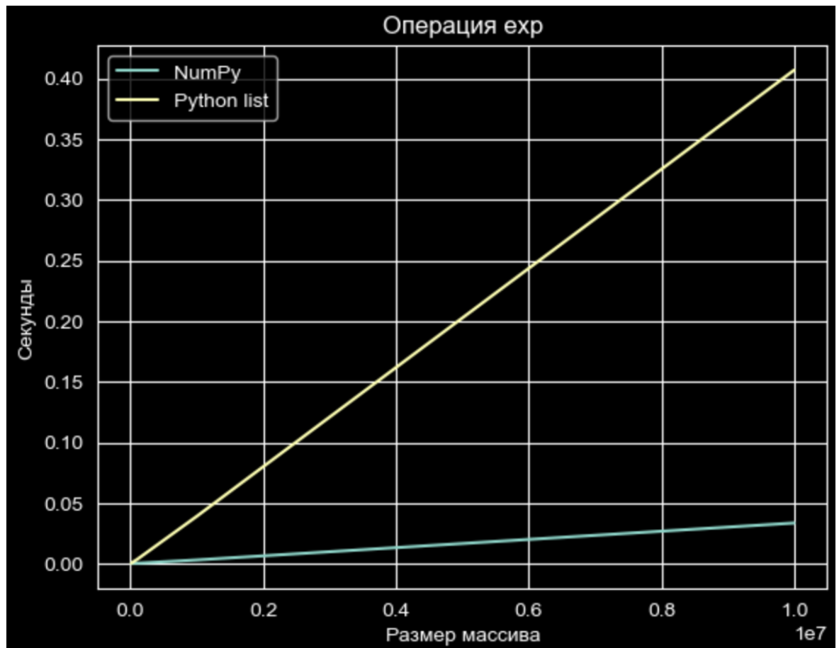
Рисунок 8 – График зависимости времени выполнения операции exp от размера массива
