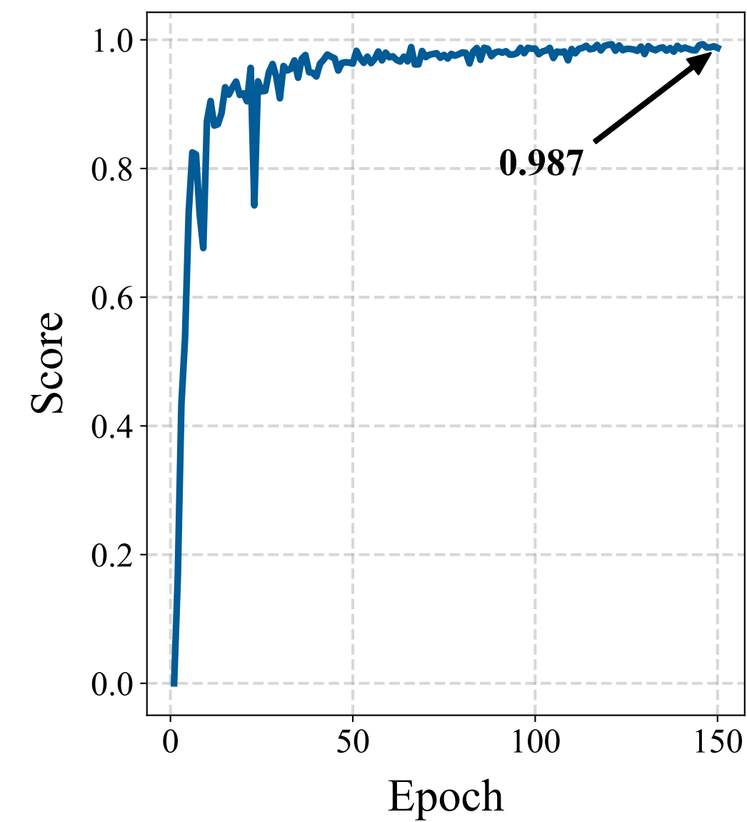
Precision (B)
