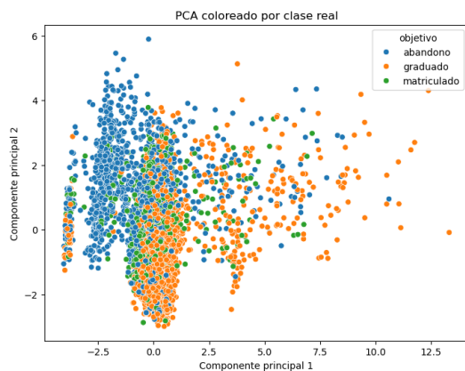
Figura 4. PCA coloreado por clase
