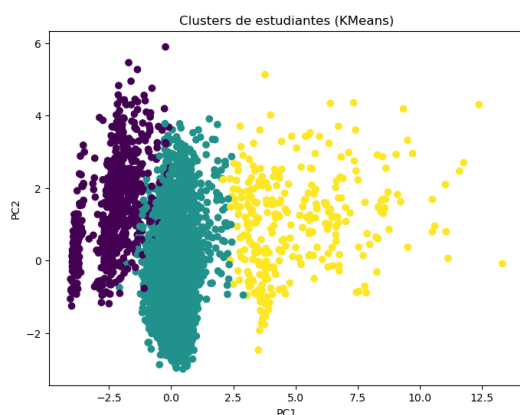
Figura 6. Clusters de estudiantes
