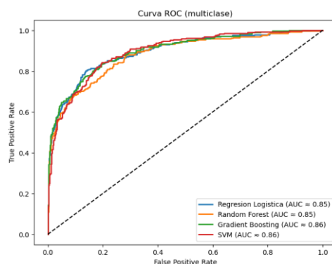
Figura 2. Curva ROC de los modelos
