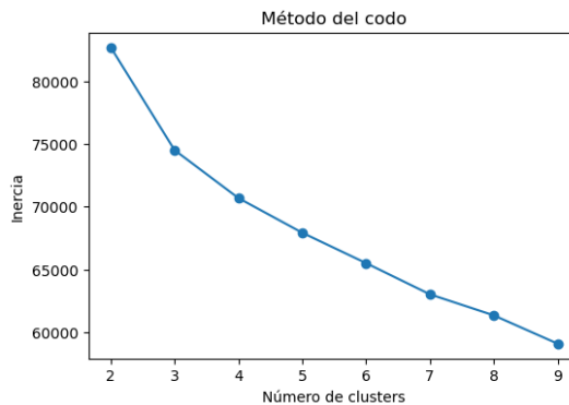
Figura 5. Método del codo
