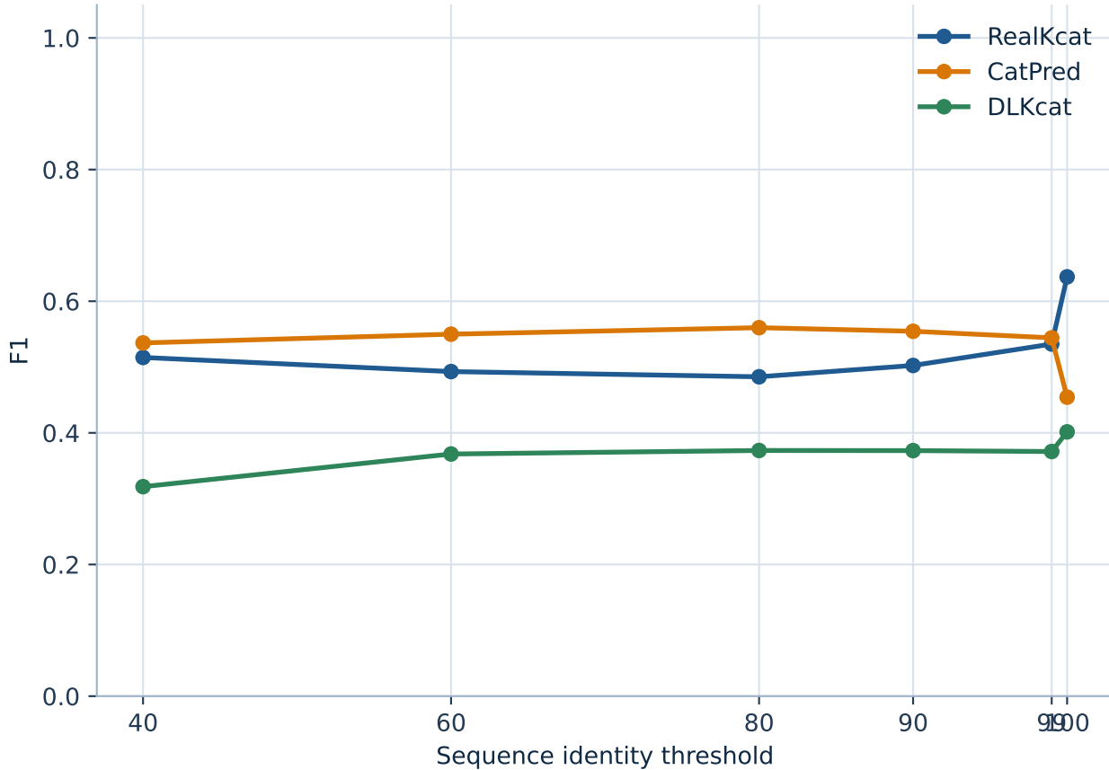
Fold 5 Sequence-Identity Benchmark: F1
