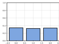
(d) \tau = 100
