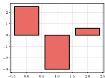
(a) Logits
