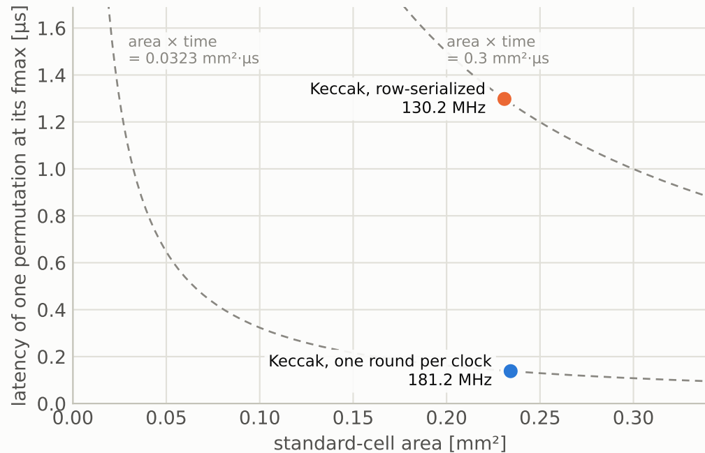
(b) Keccak-f[1600]
