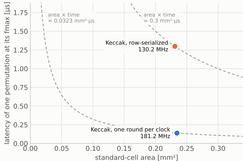
(b) Keccak-f[1600]
