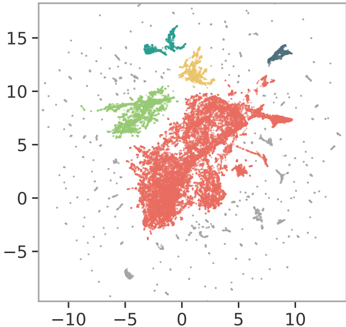
Aedes spp. - UMAP
