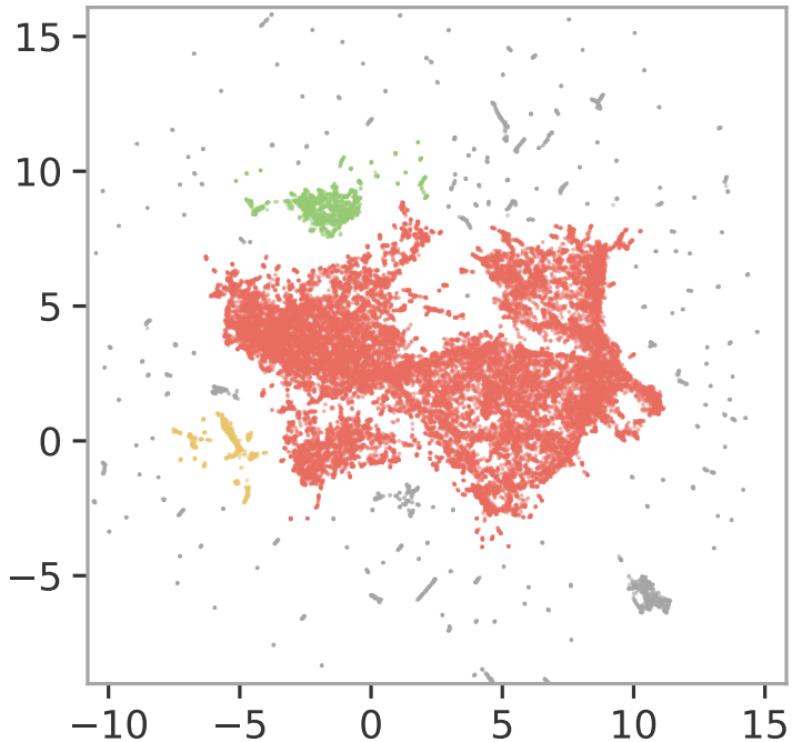
Drosophila spp. - UMAP
