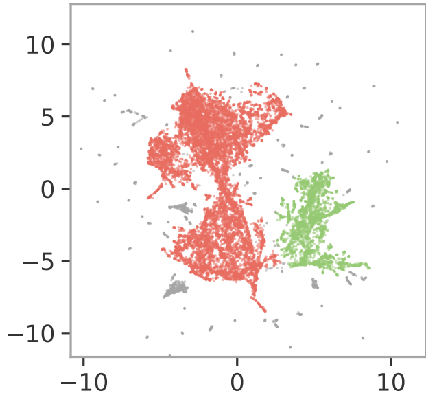
Ae. aegypti - UMAP
