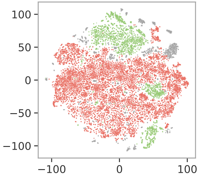
Ae. aegypti - t-SNE
