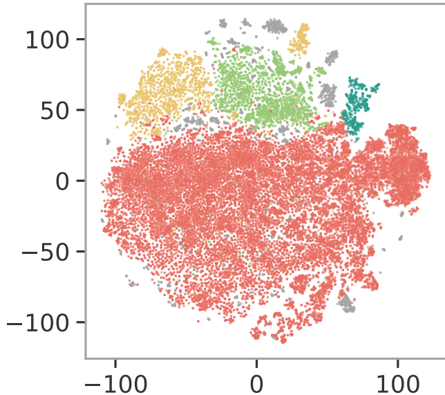
Pentatomidae spp. - t-SNE
