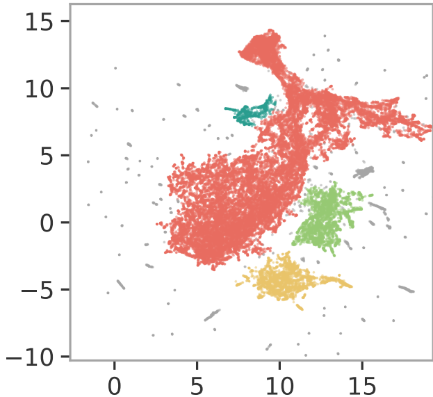
Pentatomidae spp. - UMAP
