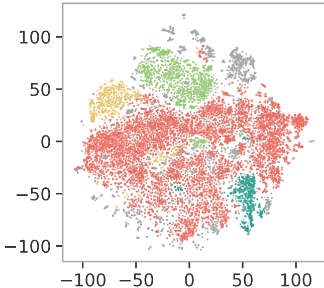
D. suzukii - t-SNE
