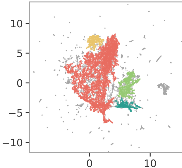
D. suzukii - UMAP
